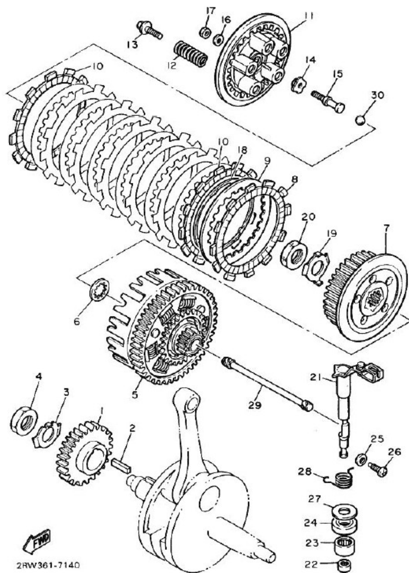
Abbg 13 KUPPLUNG
